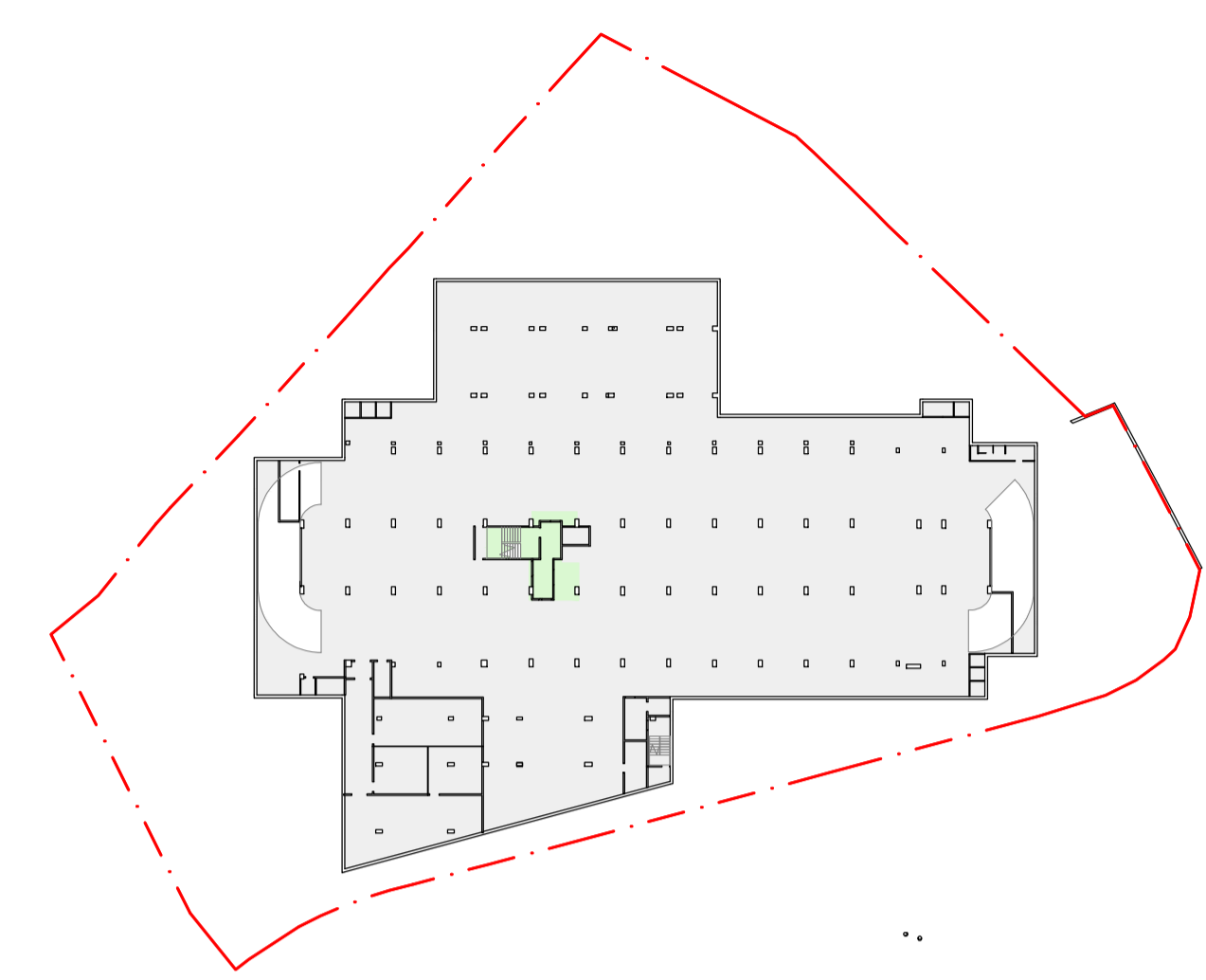
PLANTA SOTERRADA 3
