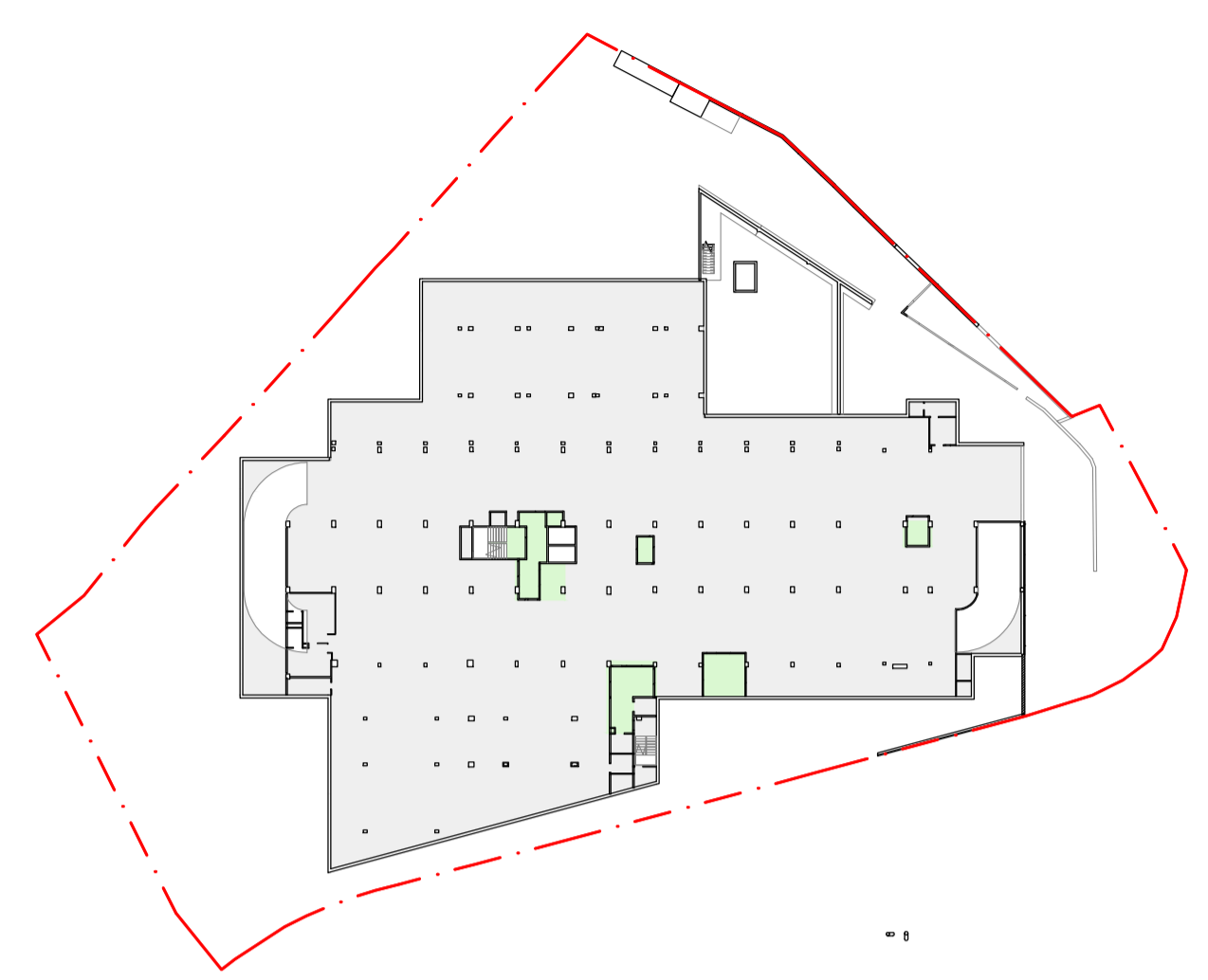
PLANTA SOTERRADA 1
